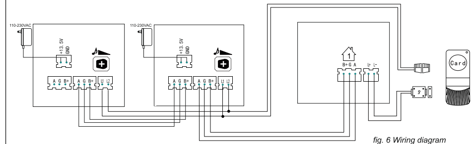
fig. 6 Wiring diagram
