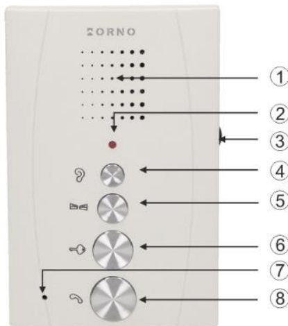
rys. 1 Budowa unifonu
