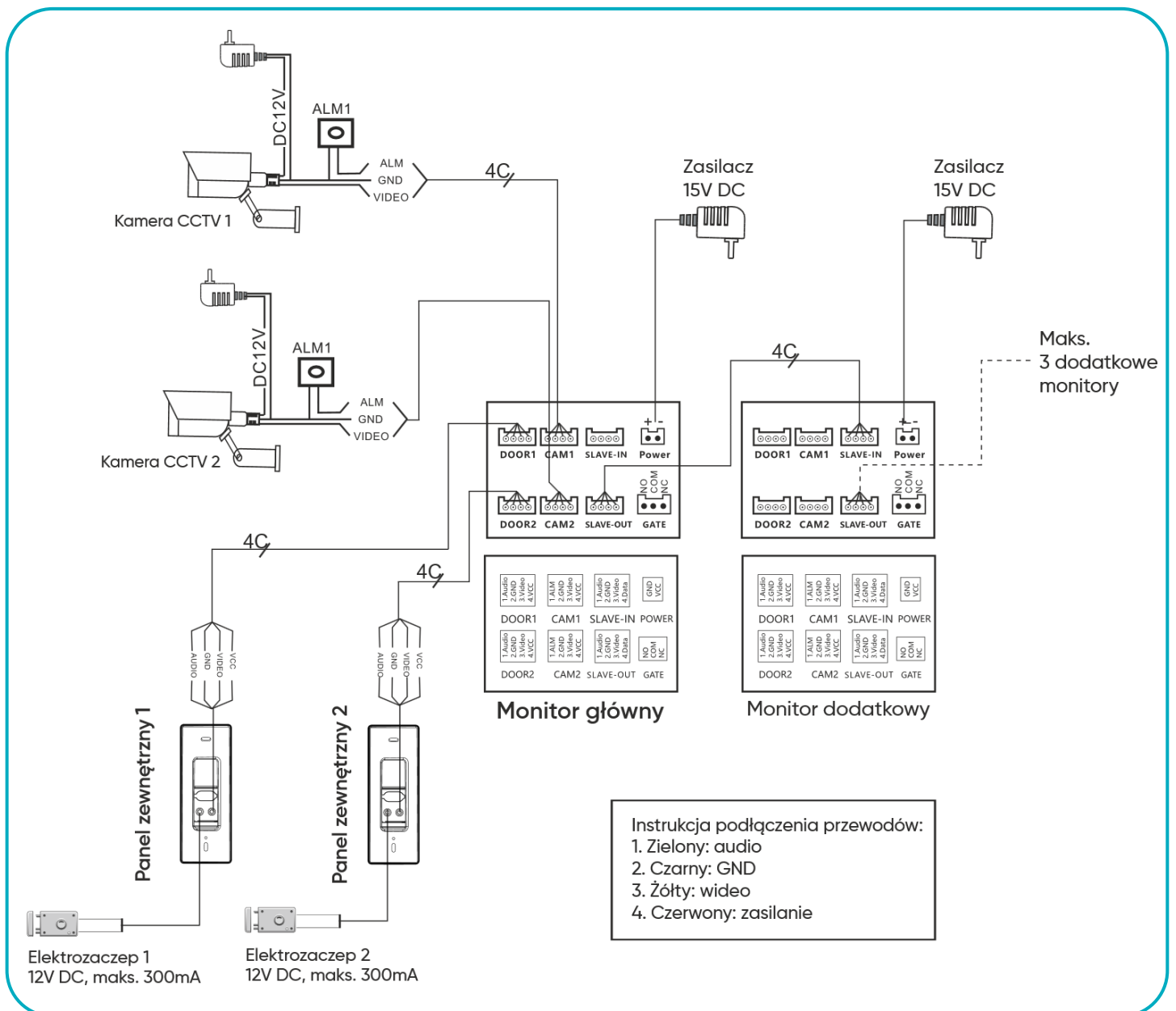
rys. 5 Schemat podłączenia
