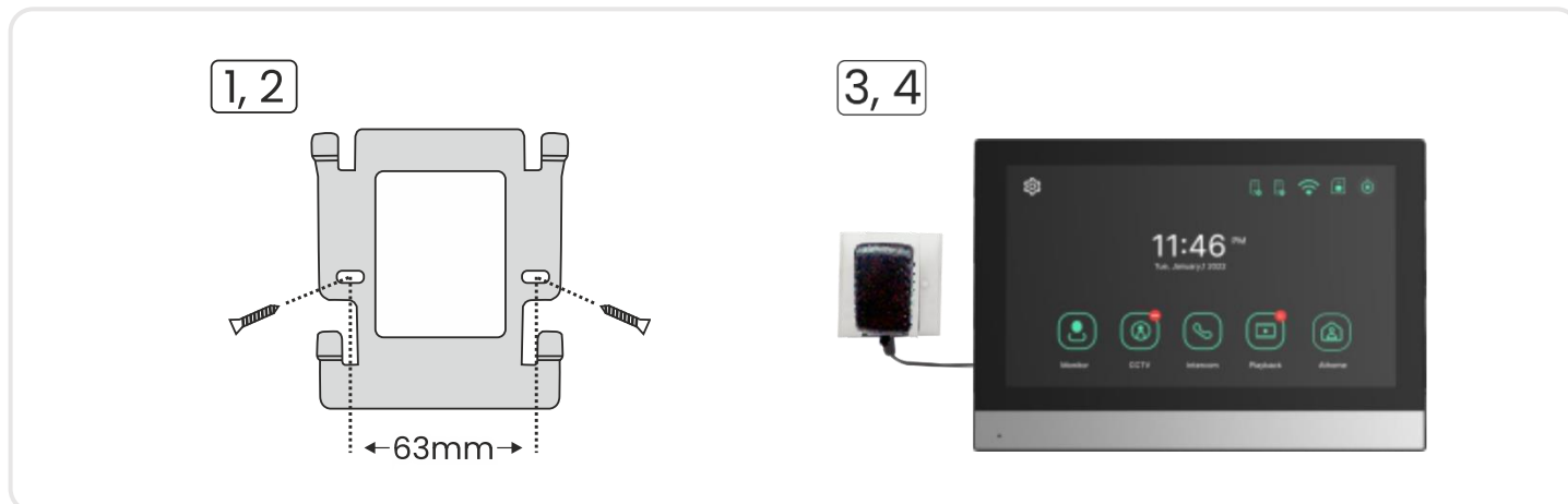
rys. 2 Montaż monitora
