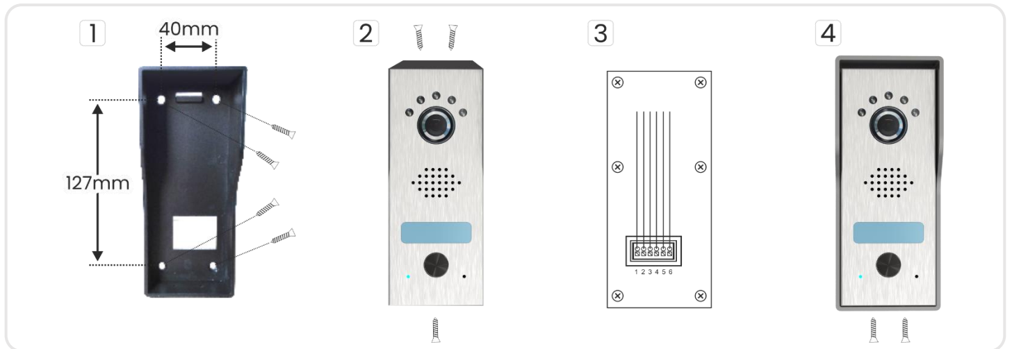
rys. 4 Montaż panelu zewnętrznego
