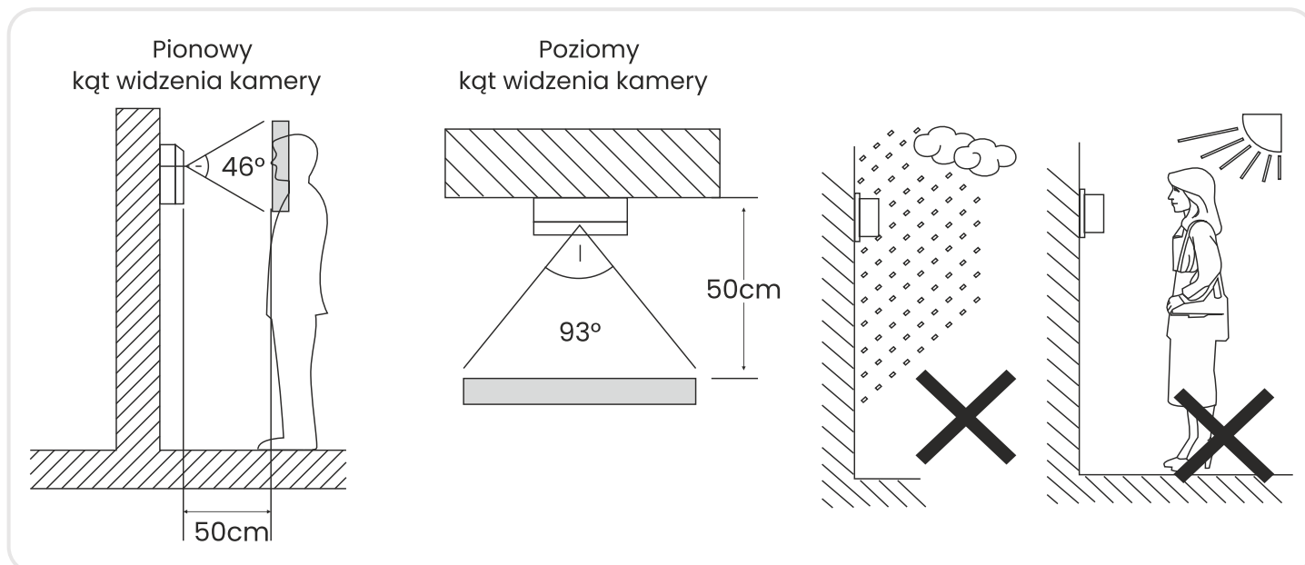
rys. 3 Umieszczenie panelu zewnętrznego
