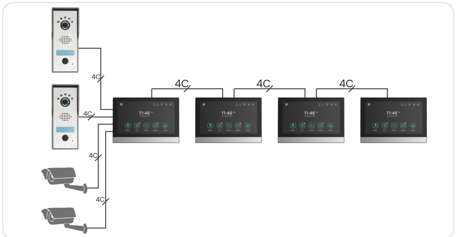
rys. 5 Schemat podłączenia
