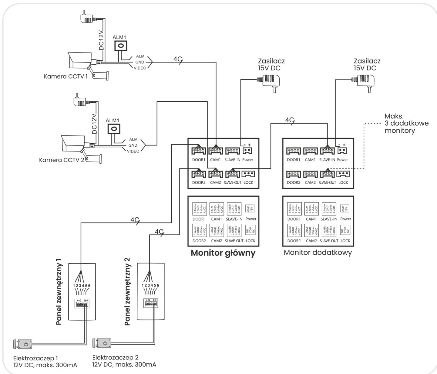
rys. 6 Schemat podłączenia
