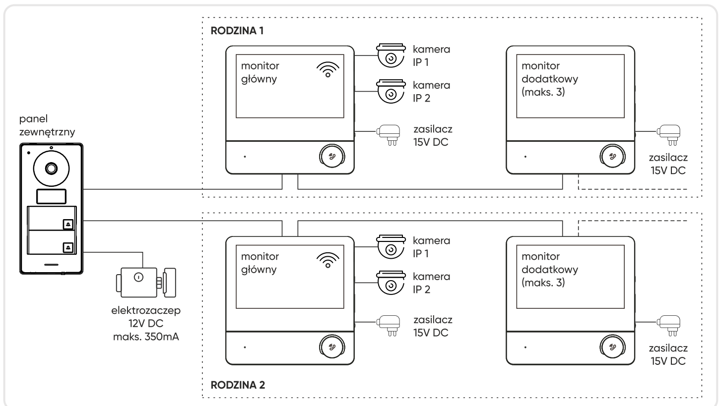
rys. 7 Schemat podłączenia
