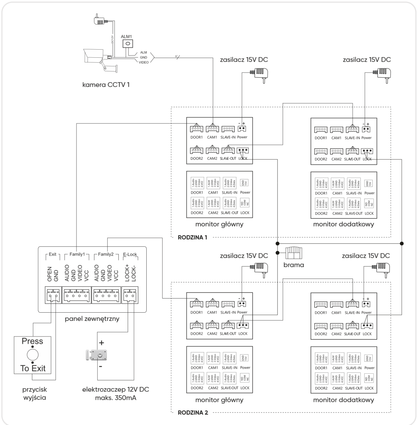
rys. 8 Schemat podłączenia
