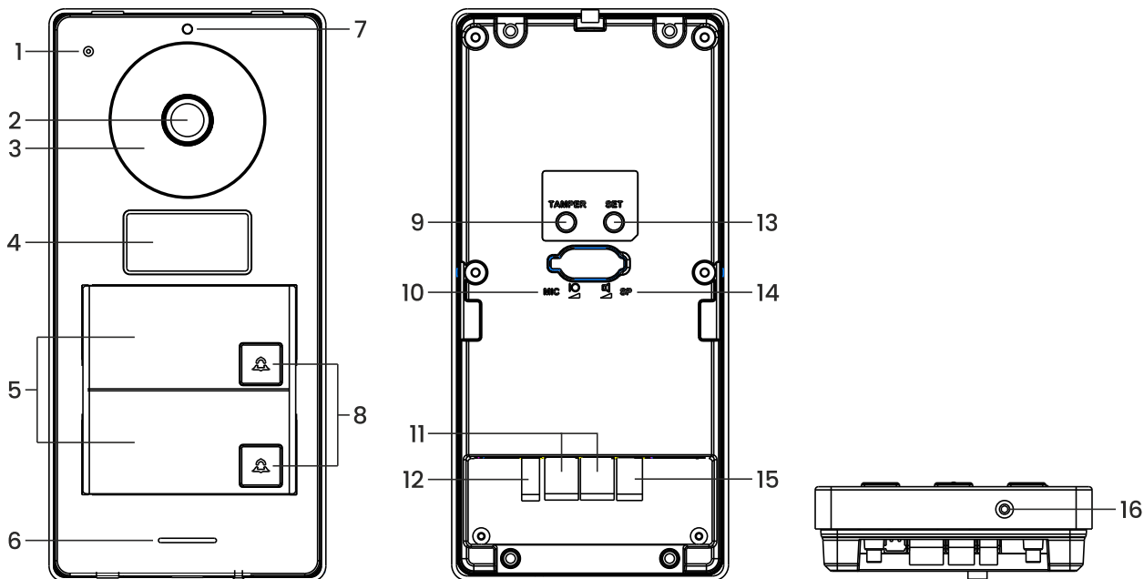
rys. 2 Budowa panelu zewnętrznego
