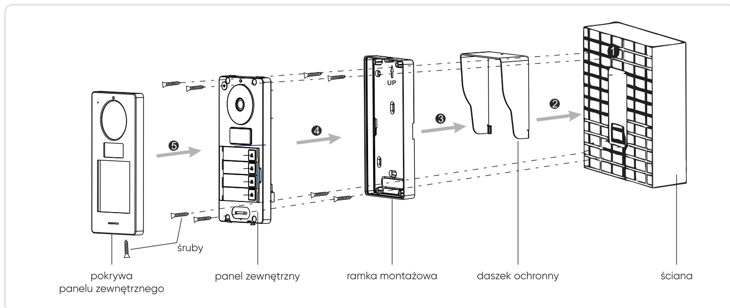
rys. 5 Natynkowy montaż panelu zewnętrznego
